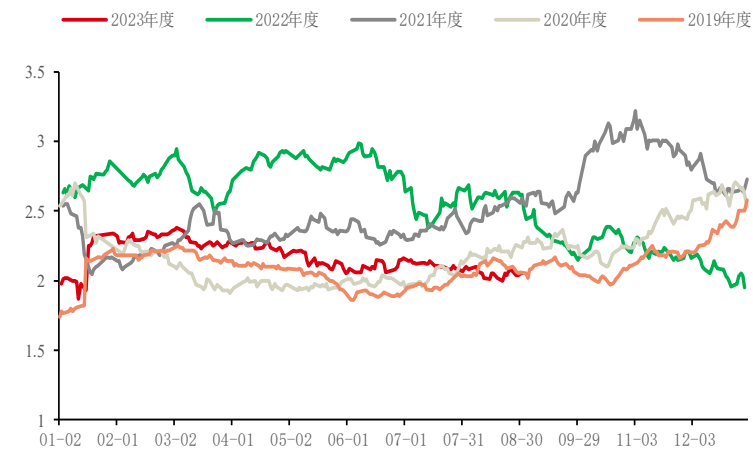
01合约油粕比
