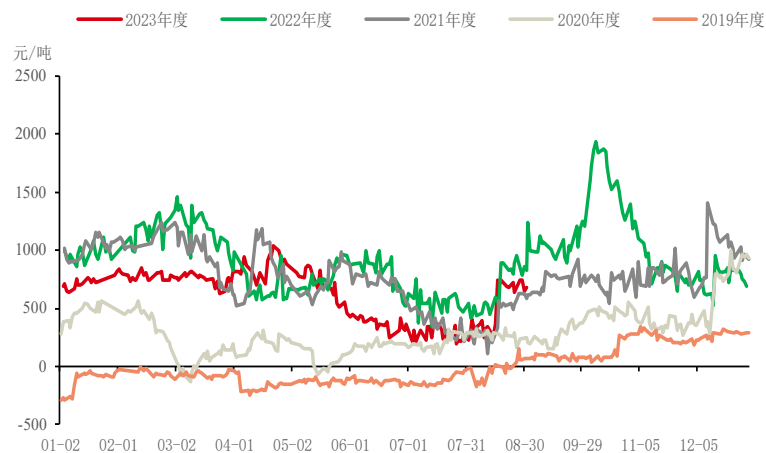
豆油基差
