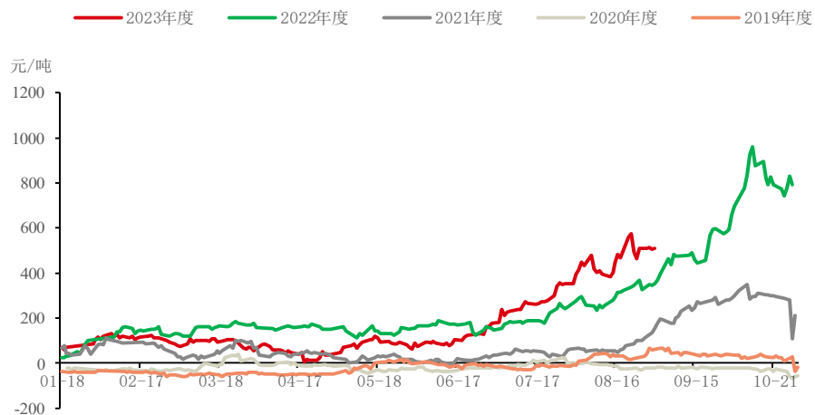
豆粕11-1价差
