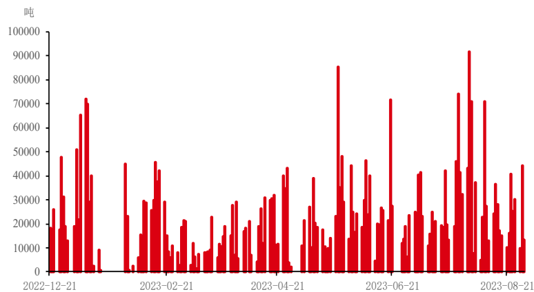
豆油成交量
