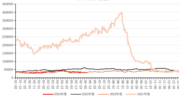
焦炭持仓量
